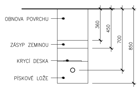
DETAIL ROZVODU V CHODNIKU KÓTY V MM
